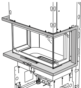
Inbouwkader 211-213
